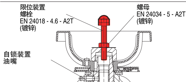
限位装置 + 自锁装置 ASTRA-Plus DN 15 - 150
