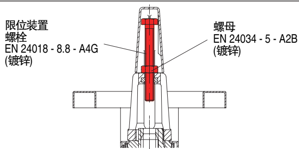
限位装置 ASTRA DN 15 - 200
