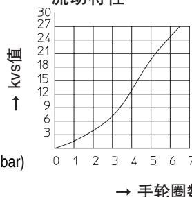
流动特性
