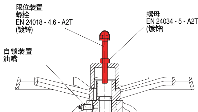
限位装置 + 自锁装置 ASTRA DN 250 - 400 ASTRA-Plus DN 200 - 400
