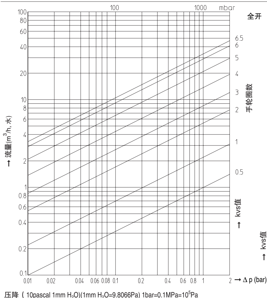
流动特性
